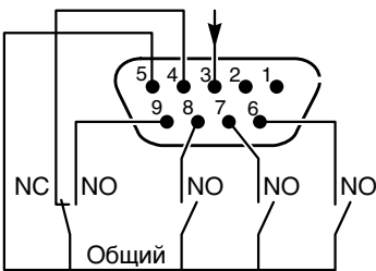
Рисунок 36. Коммуникационный порт
