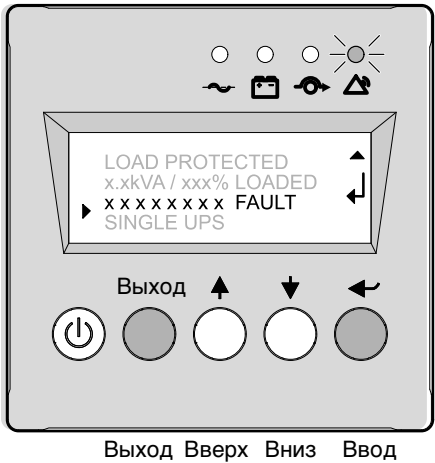
Рисунок 43. Светодиодный индикатор
