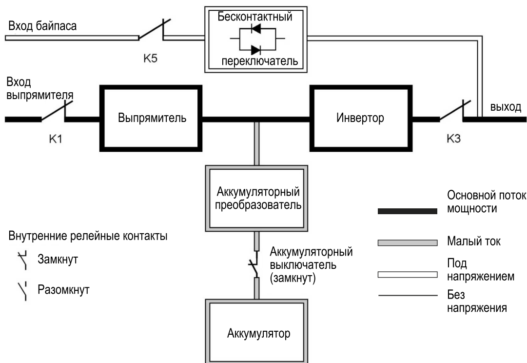
Рис. 2-3: Путь прохождения тока через ИБП в режиме двойного преобразования
