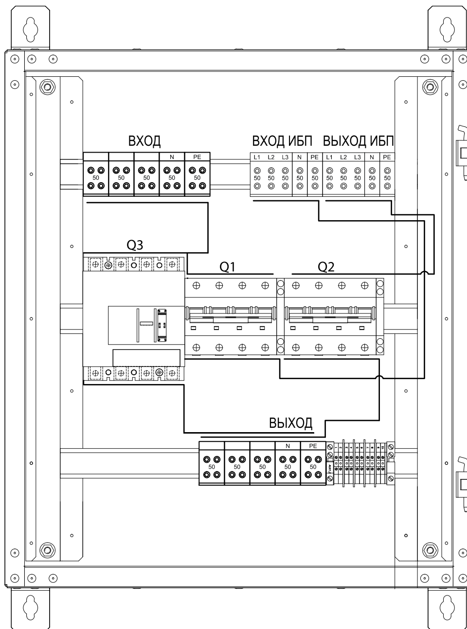
Рис. 5-4: Сборочный чертеж MBS с тремя выключателями
