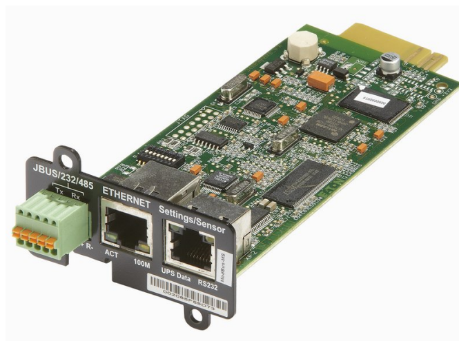
Рис. 6-5: Сетевая карта и карта MODBUS - MS
