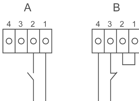
Рис. 4-4: Соединения выключателя ЕРО
