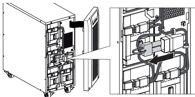
Рисунок 28. Отсоединение внутренних аккумуляторных батарей ИБП.
