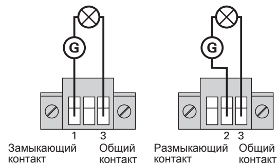
Рисунок 26. Пример соединения стандартного релейного порта с лампочкой.
