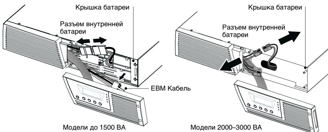
Рисунок 24. Отключение внутренних батарей ИБП (показано без EBM)
