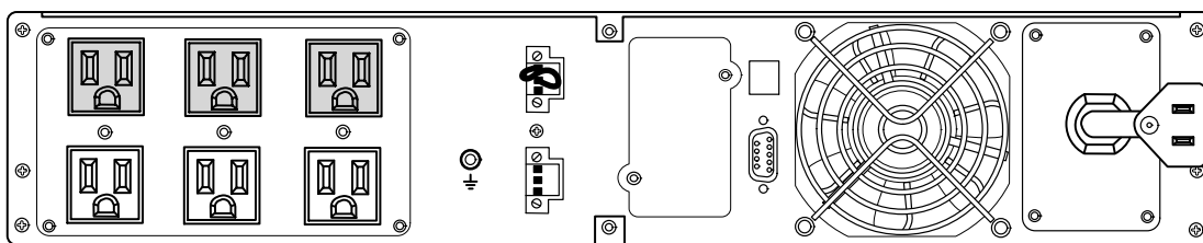
Рисунок 33. Модель PW9130L1500R-XL2U
