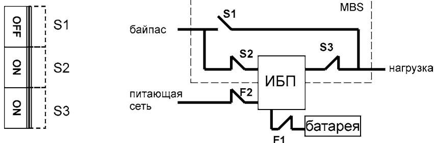
Рисунок 17 Нормальное положение выключателей MBS (ИБП питает нагрузку).
