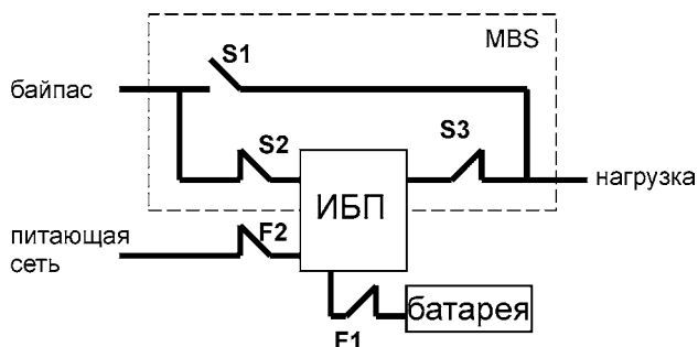
Рисунок 16 Нормальное положение выключателей MBS.
