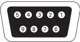
Рисунок 22. Коммуникационный порт RS-232 (разъем DB-9).
