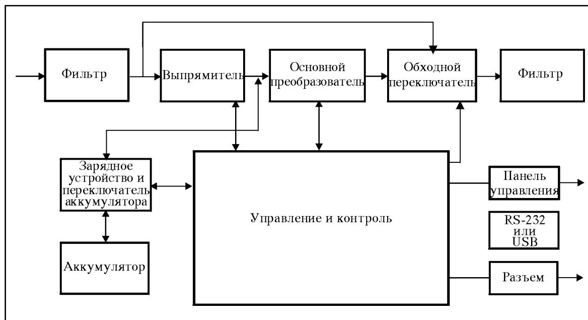
Рис. 1. Блок-схема ИБП
