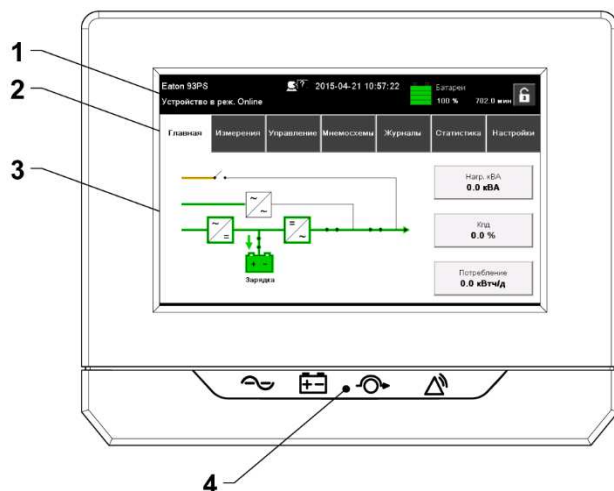
Рисунок 33. Элементы дисплея
