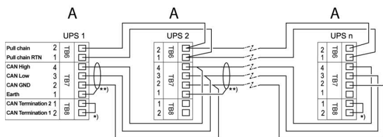
Рисунок 22. Проводка для сети CAN и параллельного монтажа для системы ИБП с параллельным подключением без выходных выключателей модулей
