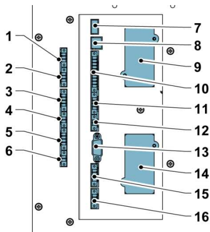
Рисунок 23. Интерфейсы связи ИБП Eaton 93PS 8-20 кВт
