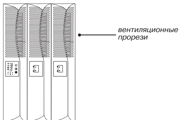
Рисунок 9. Вертикальная установка трех модулей
