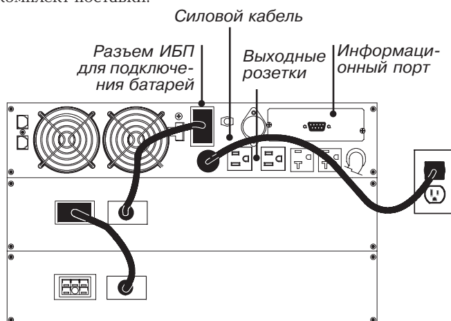
Рисунок 15. Пример подключение ИБП (Модель 120В)
