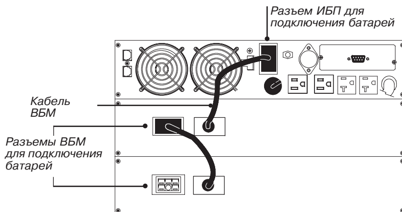
Рисунок 11. Подключение ВБМ (на примере модели ИБП 120В)
