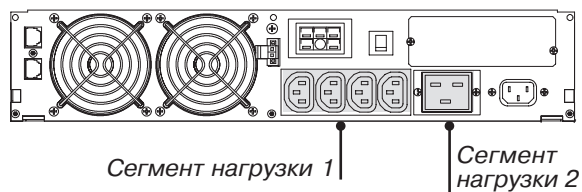
Рисунок 37. Сегменты нагрузки ИБП для моделей 208В/230В
