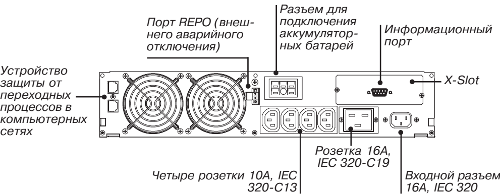
Рисунок 23. 2500/3000 ВА, 208В Задняя панель
