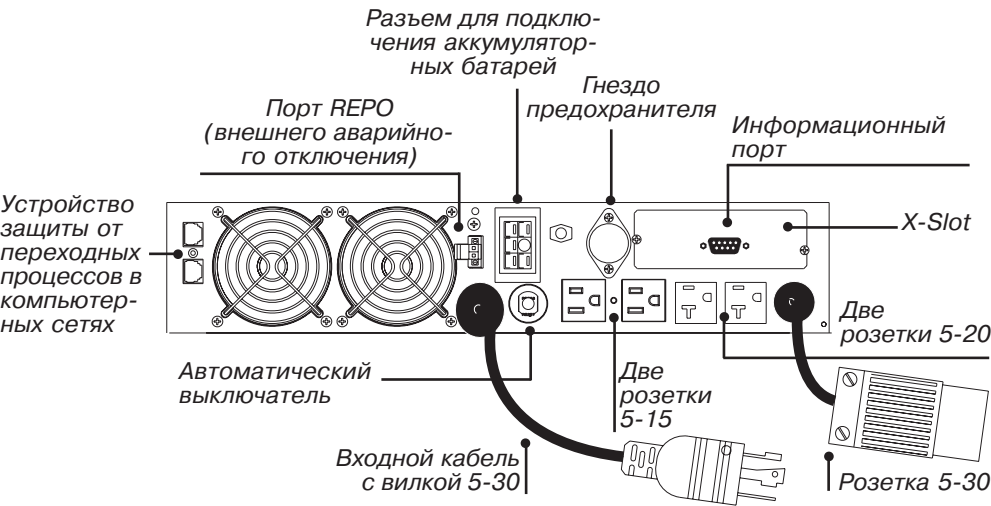
Рисунок 22. 2500/3000 ВА, 120В Задняя панель
