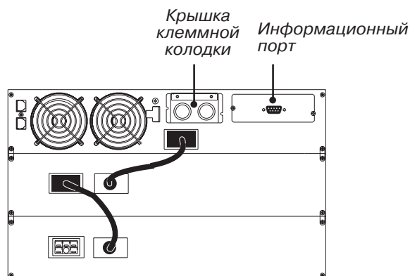
Рисунок 17. Пример фиксированного подключения ИБП
