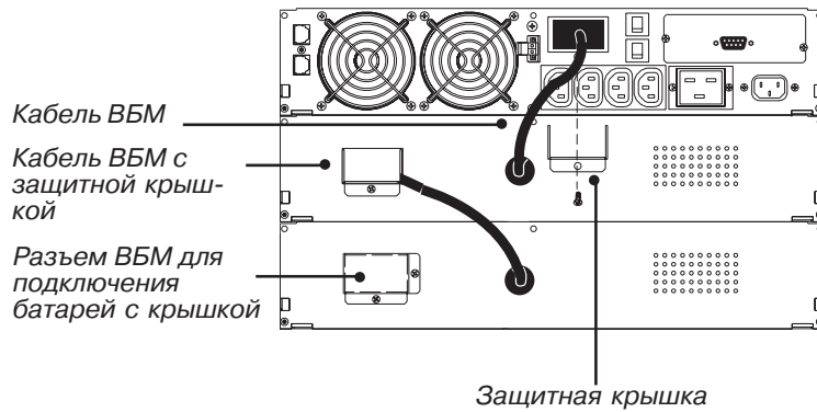
Рисунок 14. Подключение ВБМ для моделей 230В
