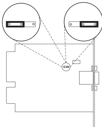
Рисунок 34. Перемычка релейного контакта На Байпасе
