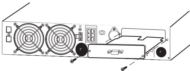
Рисунок 33. Снятие однопортового модуля
