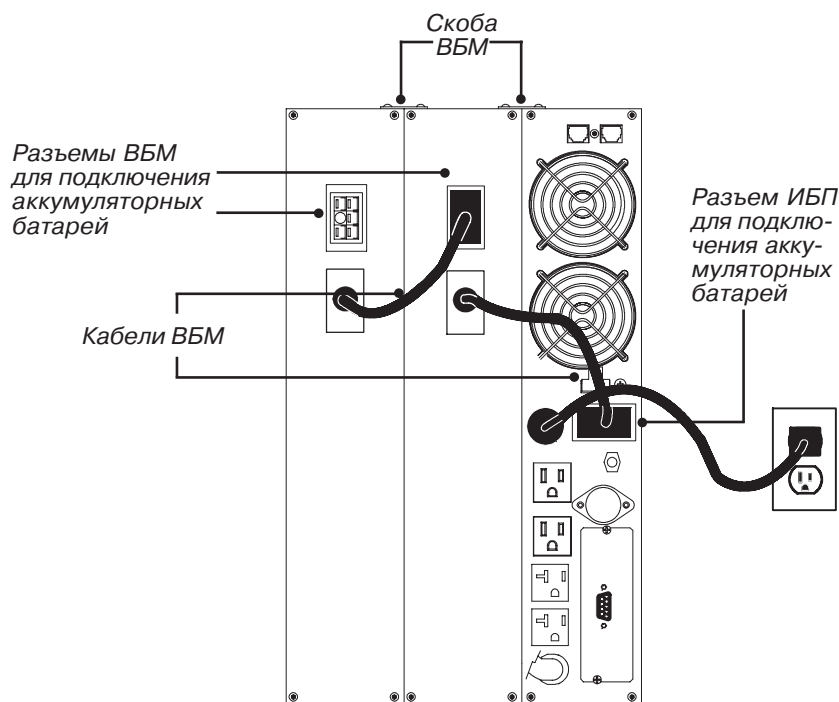
Рисунок 38. Подключение ВБМ (модель 120В)
