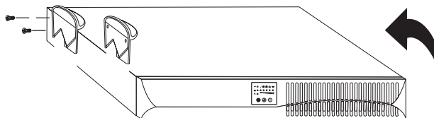
Рисунок 6. Установка подставок ИБП с двумя модулями.
