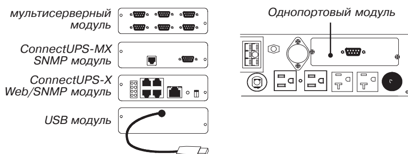
Рисунок 31. Дополнительные X-Slot модули
