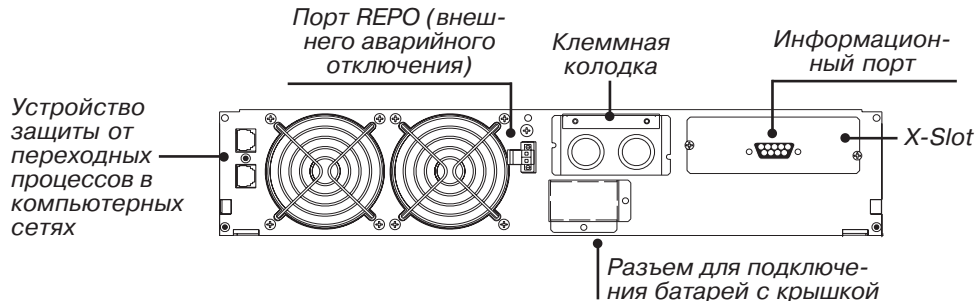
Рисунок 26. 2500/3000 ВА, 230В Задняя панель для фиксированного подключения
