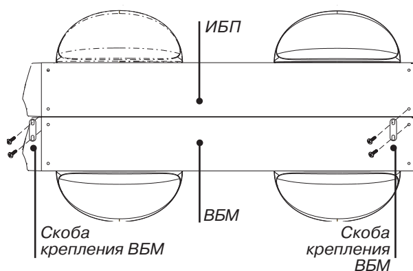
Рисунок 10. Установка скоб крепления ВБМ (Вид сверху с подставками)
