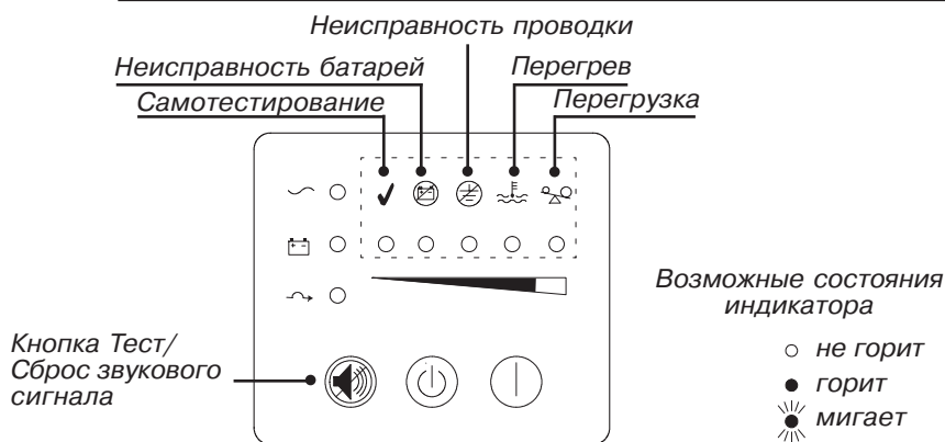
Рисунок 39. Индикаторы неисправности
