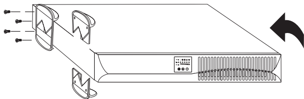
Рисунок 4. Установка подставок на одиночный ИБП
