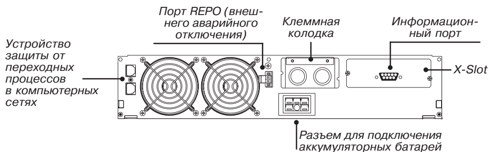
Рисунок 25. 2500/3000 ВА, 208–240В Задняя панель для фиксированного подключения
