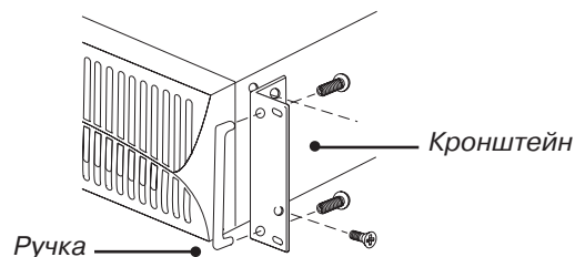
Рисунок 2. Установка кронштейнов
