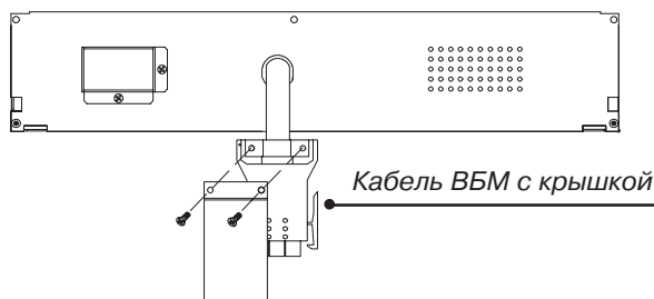
Рисунок 13. Защитная крышка кабеля ВБМ (только у ВБМ 230В)
