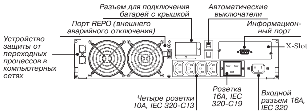
Рисунок 24. 2500/3000 ВА, 230В Задняя панель
