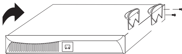
Рисунок 7. Установка подставок на ВБМ
